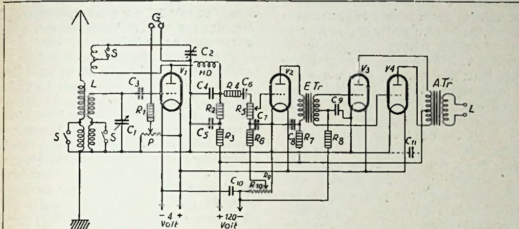
Fig. 1. Toestel zonder hfr. trap.
