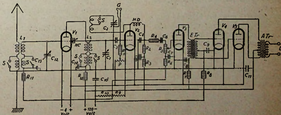
Fig. 2. Toestel met hoogfrequenttrap.
